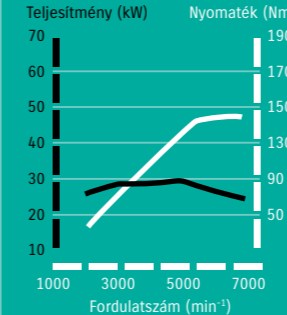
1 literes motor teljesítménygörbéje (65 LE/48 kW)
